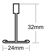
PN 400 Main Tee
