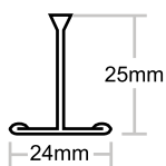
PN 401/402 Cross Tee
