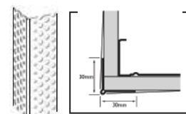
PN 300: External Angle 90° (2700 & 3000 mm)
